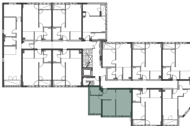
BILANS POVRŠINA: STVARNA POV.m 2 k PRODAJNA POV.m 2 ① ULAZ 6,32 1.0 6,23 ② DNEVNI BORAVAK I TRPEZARIJA 18,40 1.0 18,40 ③ SOBA 1 9,63 1.0 9,63 ④ SOBA 2 9,37 1.0 9,37 ⑤ KUPATILO 3,89 1.0 3,89 UKUPNO 47,61 47,61 KVADRATURE STANOVA SU PROJEKTANTSKE
