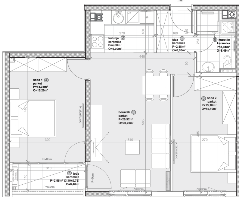
BILANS POVRŠINA: STVARNA POV.m 2 k PRODAJNA POV.m 2 ① ULAZ 2,88 1.0 2,88 ② KUHINJA 4,60 1.0 4,60 ③ DNEVNI BORAVAK I TRPEZARIJA 20,92 1.0 20,92 ④ SOBA 1 14,04 1.0 14,04 ⑤ SOBA 2 13,10 1.0 13,10 ⑥ KUPATILO 3,94 1.0 3,94 ⑦ LOĐA 3,40 0.75 2,55 UKUPNO 62,88 62,03 KVADRATURE STANOVA SU PROJEKTANTSKE
